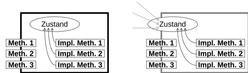
Objekt als Implementierung eines ADT
